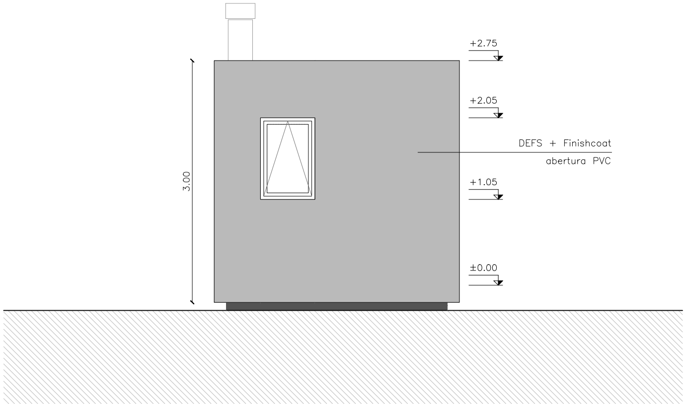
FACHADA OESTE
