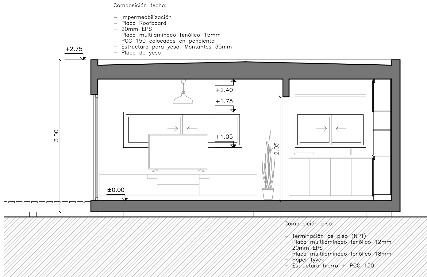
CORTE AA
