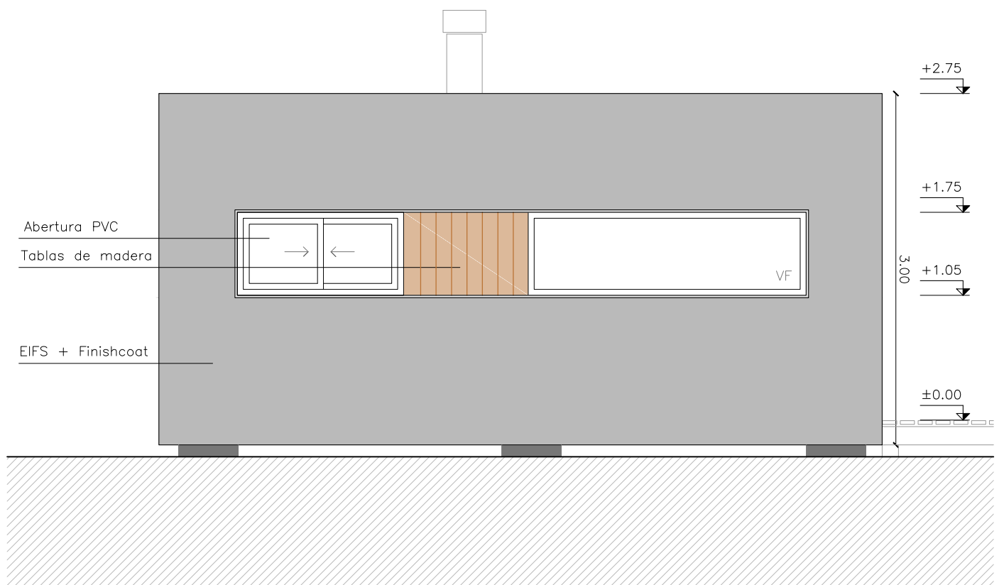
FACHADA NORTE
