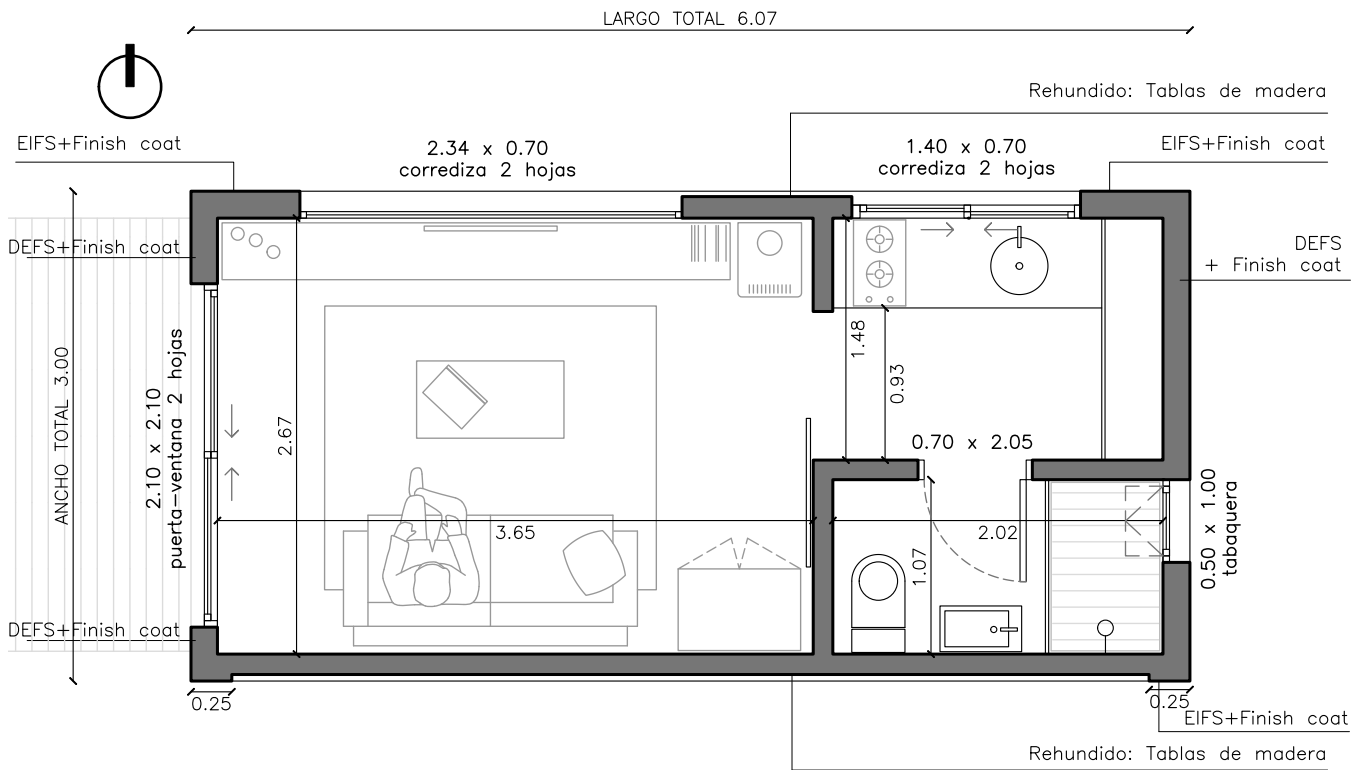
PLANTA
