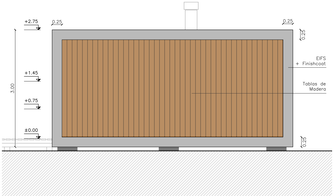
FACHADA SUR
