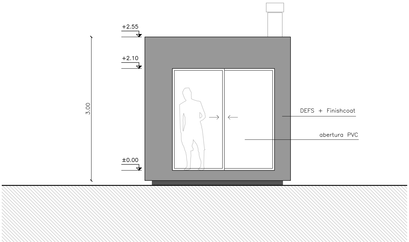
FACHADA ESTE
